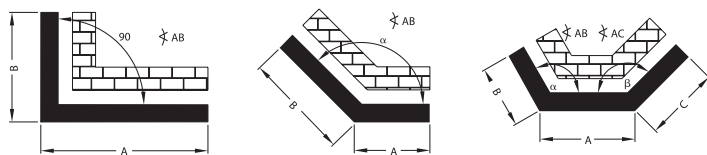
внешний угол 90^\circ
