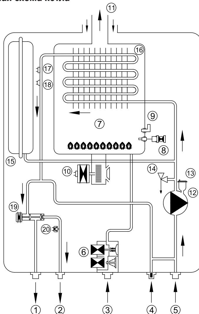
Рисунок 3. Функциональная схема котла.
