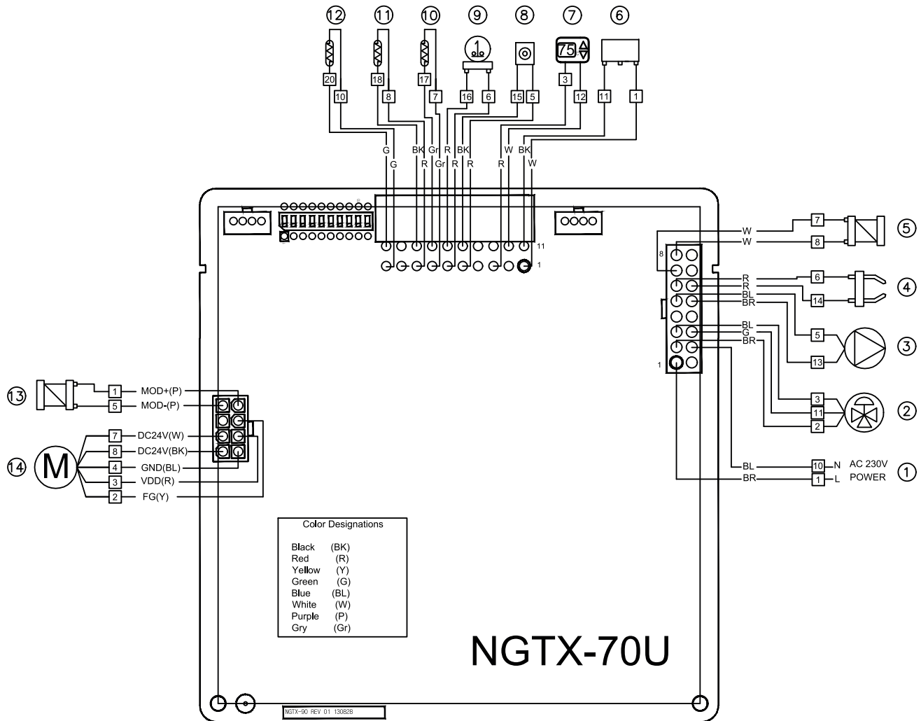
Рисунок 16. Схема электрическая.
